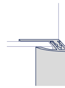
Click-Abschlussprofil aus Aluminium (Ref. 06430001)
