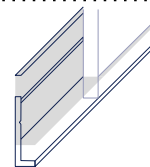
Boden-Abschlussprofil (Anfangsprofil) aus Aluminium (Ref. 06520001)
