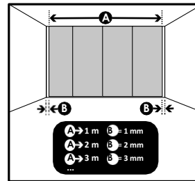
DEHNUNGSFUGENABSTAND
